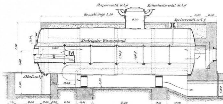
Abb. 6. Längenschnitt C-D durch den Kessel. 1:70.
