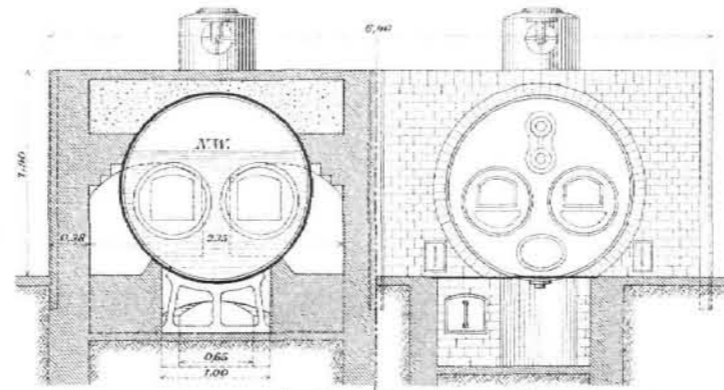
Abb. 7. Querschnitt E-F-G durch die Kesselanlage.
