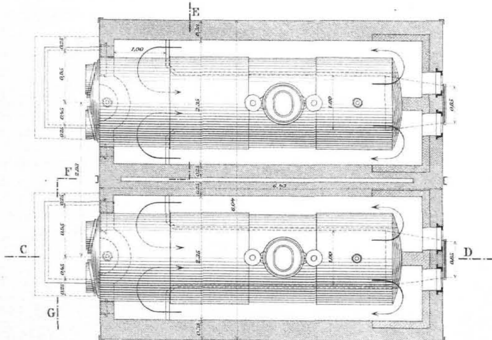
Abb. 8. Grundriß der Kesselanlage. 1:70.
