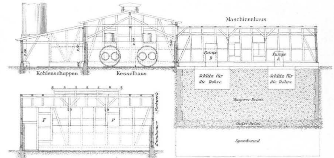
Abb. 3. Längenschnitt durch das Kesselhaus. 1:175.
